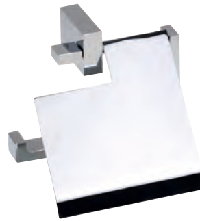
WC-papír tartó Toilet paper holder without cover 128×135×50 mm
